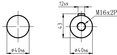
轴型式 S1
